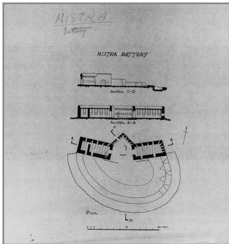
Disinn Nru 1
