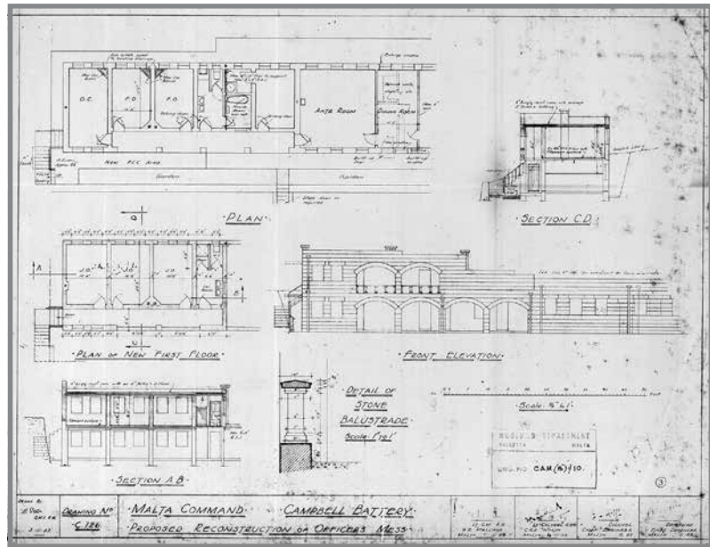
Pjanta Nru 3
